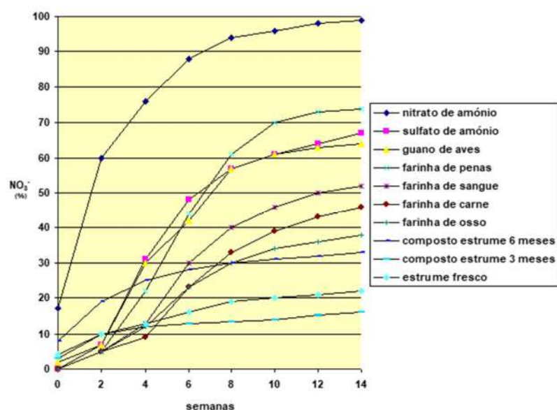
Figura 7.4 – Quantidades libertadas de azoto nítrico (nitratos) para a cultura a partir de diferentes adubos minerais (nitrato e sulfato de amónio), de adubos orgânicos simples (guano de aves marinhas, farinha de penas, farinha de carne e farinha de osso) e de corretivos orgânicos (estrume de vaca fresco e composto com 3 e 6 meses de compostagem feito com o mesmo estrume de vaca).
